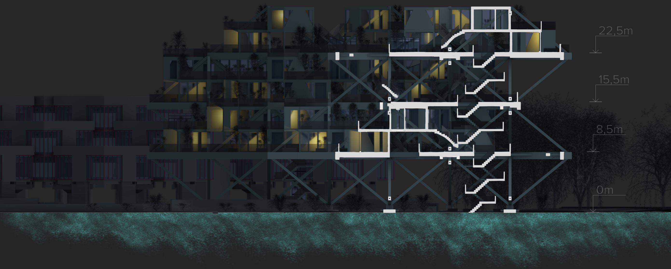
Podélný řez B 1:250
