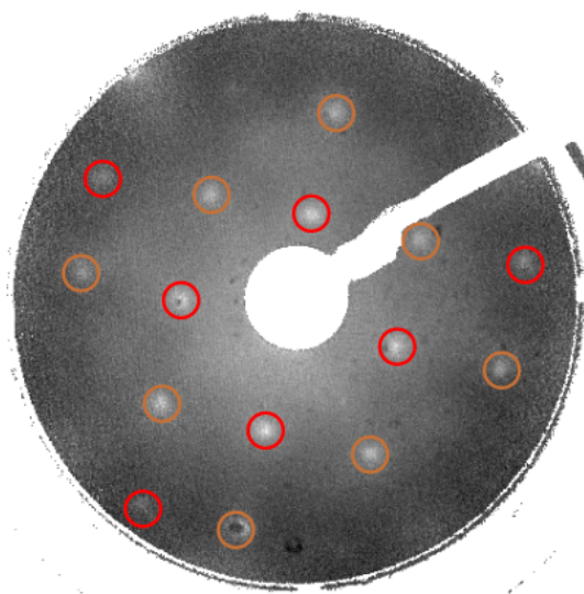
Obrázek 4.10: Difrakční obrazec FeRh po druhém odprašování a žíhání, E = 100 eV. Reciproká mřížka FeRh je značena hnědě, rekonstrukce (\sqrt{2} \times \sqrt{2})R45^\circ je značena červeně.
