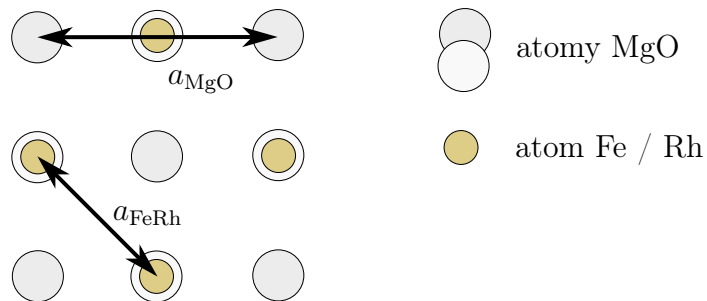
Obrázek 3.3: Epitaxní růst FeRh na krystalu MgO. Protože roviny (001) v FeRh jsou alternující vzájemně posunuté monovrstvy železa a rhodia, může růst začít kteroukoliv z nich.
