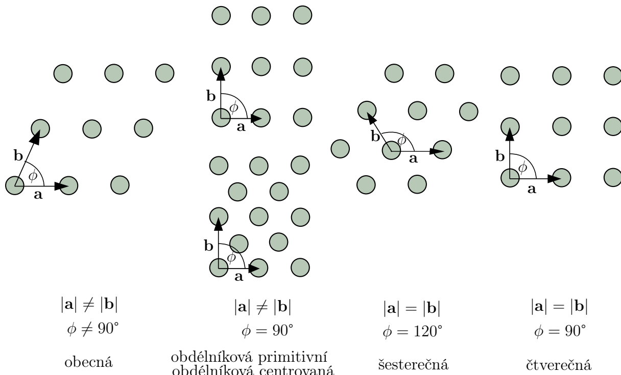
Obrázek 2.1: Rovinné elementární buňky.
