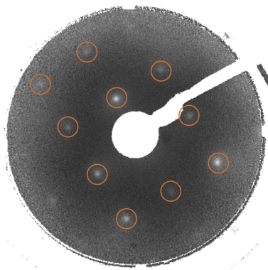
Obrázek 4.9: Difrakční obrazec FeRh po jemném odprašování a žíhání, hnědě jsou zvýrazněny body reciproké mřížky FeRh, E = 160 eV.
