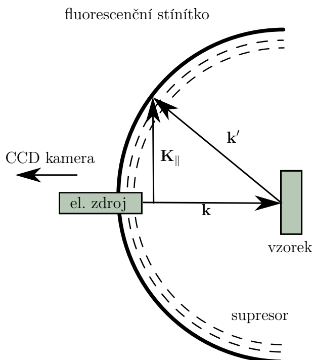
Obrázek 4.1: Schematické znázornění přístroje LEED.
