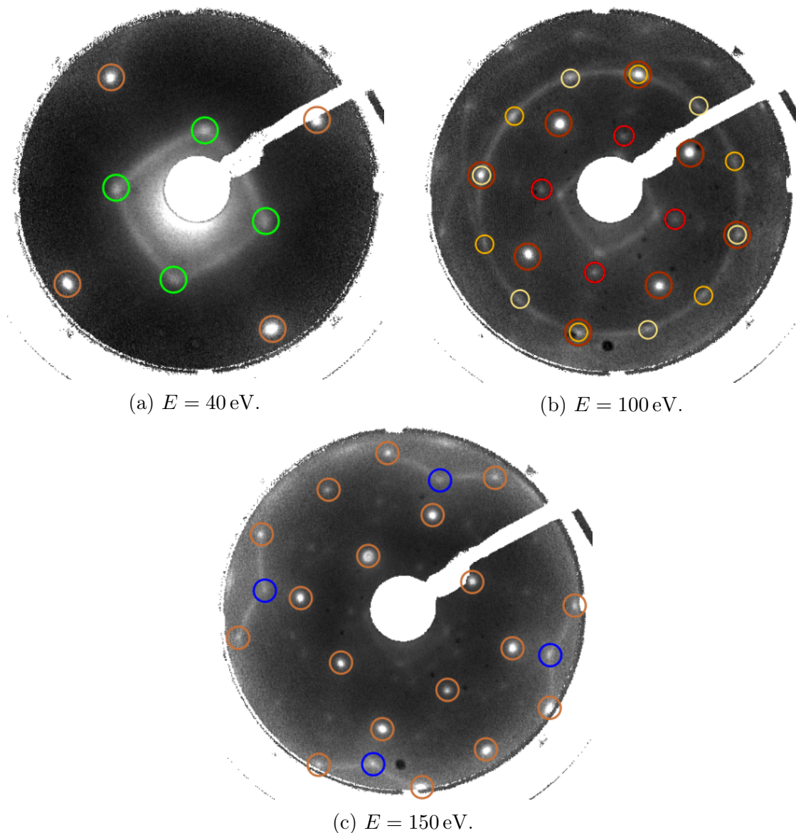
Obrázek 4.11: Snímky difrakce na povrchu FeRh po prvním dlouhém žíhání. Zelenou a modrou barvou jsou značeny struktury původem připisované moiré grafenu a FeRh, hnědě je značena reciproká mřížka FeRh, červeně rekonstrukce (\sqrt{2} \times \sqrt{2})R45^\circ . Světle a tmavě žlutou jsou zvýrazněny dvě preferenční orientace grafenu.
