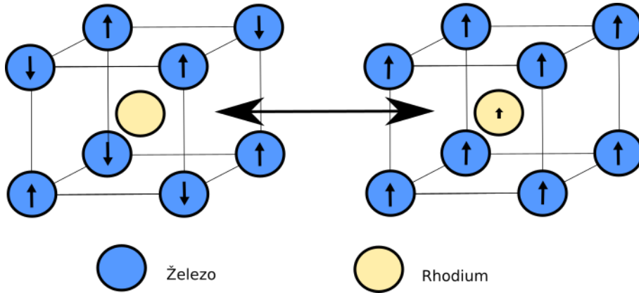
Obrázek 3.2: Elementární buňka ekviatomární slitiny FeRh a uspořádání magnetických dipólových momentů v AF a FM fázi [13].
