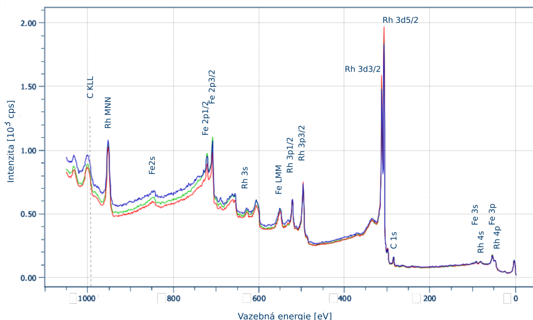
Obrázek 4.8: XPS spektrum FeRh. Modře je vyznačeno měření před prvním čištěním (po třech týdnech v UHV systému), červenou barvu má měření po prvním odprašování a žíhání. Zelenou barvou je značené měření provedené ihned po získání difrakčních obrazců obsahujících grafen, viz. Obr. 4.11
